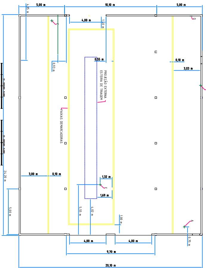
PLANTA DE LAYOUT EQUIPAMENTOS ESCALA - 1/120
